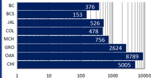
SISMOS CON M ≥ 4.5 GRADOS EN MÉXICO
