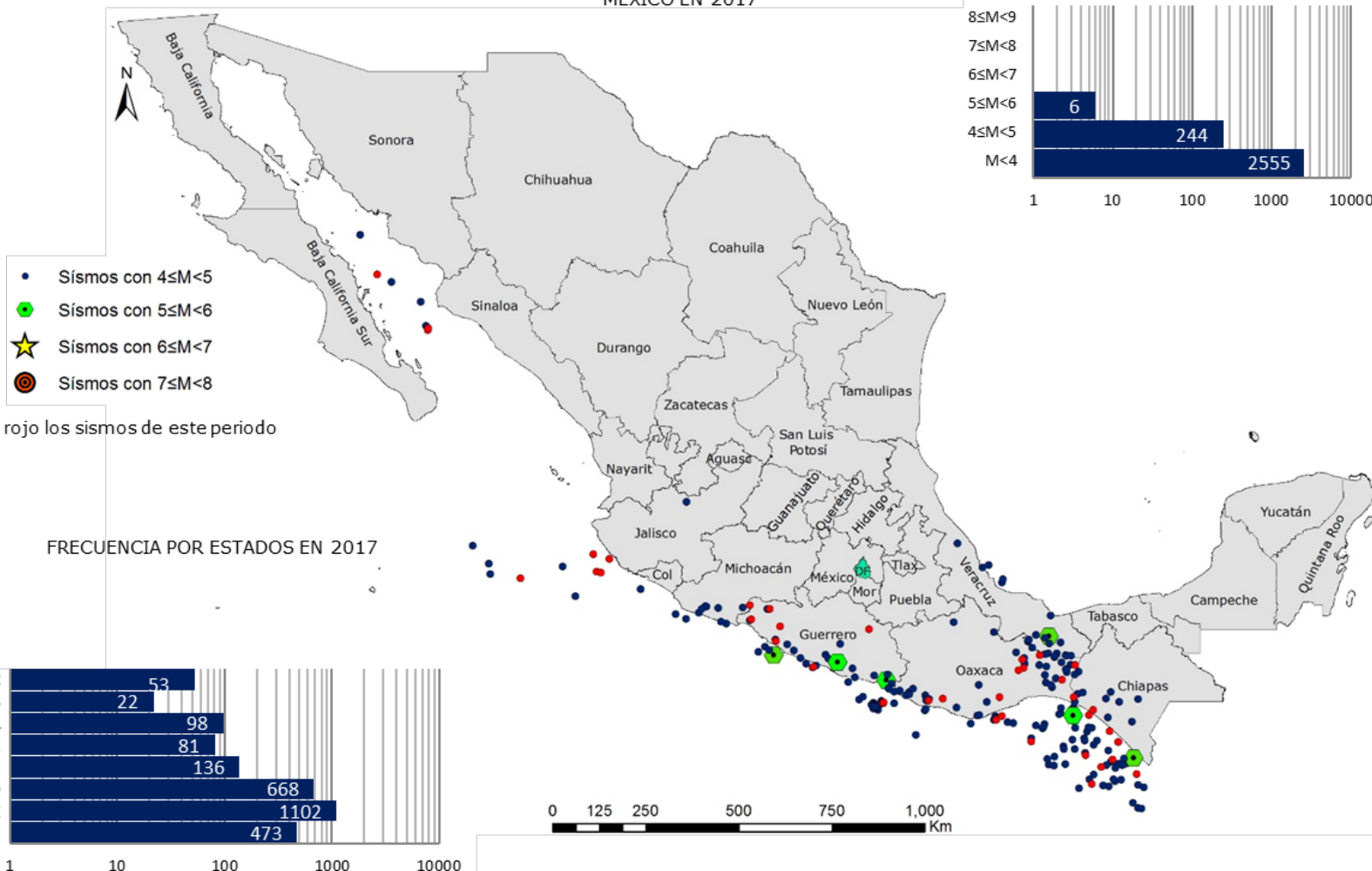
LOCALIZACIÓN DE EPICENTROS EN MÉXICO EN 2017
