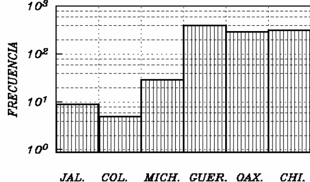
FRECUENCIA EN ZONAS DEL PACIFICO
