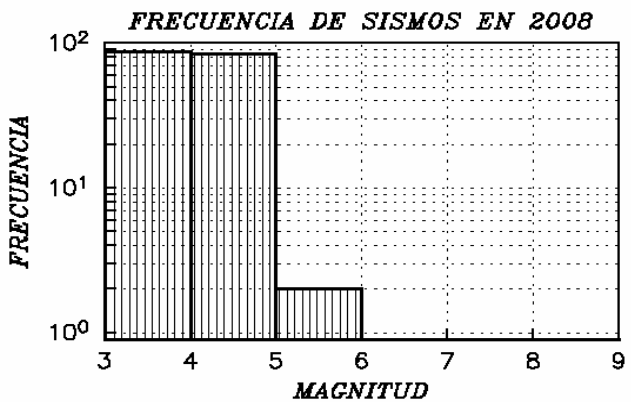
FRECUENCIA DE SISMOS EN 2008
