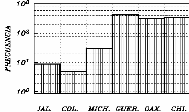
FRECUENCIA EN ZONAS DEL PACIFICO
