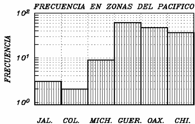
FRECUENCIA EN ZONAS DEL PACIFICO
