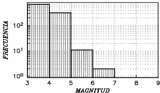
FRECUENCIA DE SISMOS EN 2008
