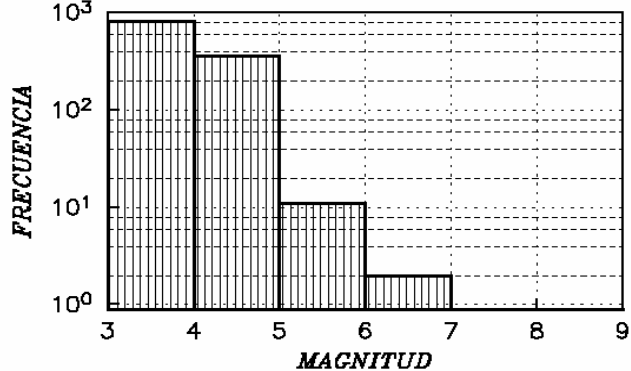
FRECUENCIA DE SISMOS EN 2008
